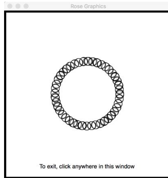
draw_cosines_and_sines()
