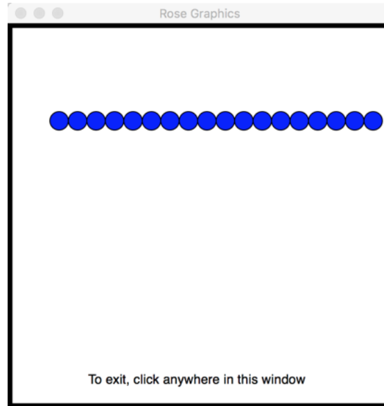
draw_circles2()
